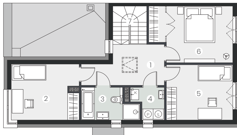
RZUT PIĘTRA
