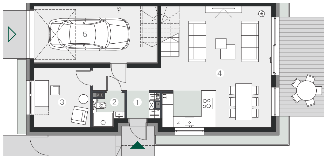
RZUT PARTERU
