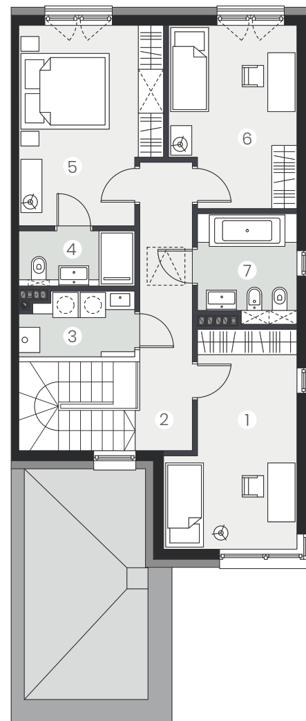
RZUT PIĘTRA
