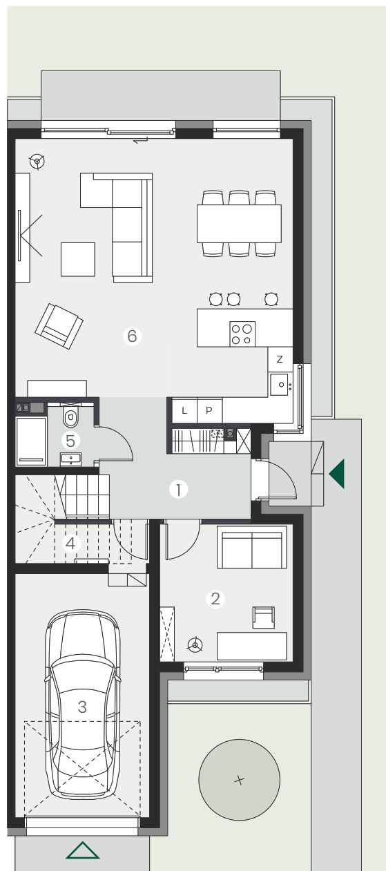
RZUT PARTERU
